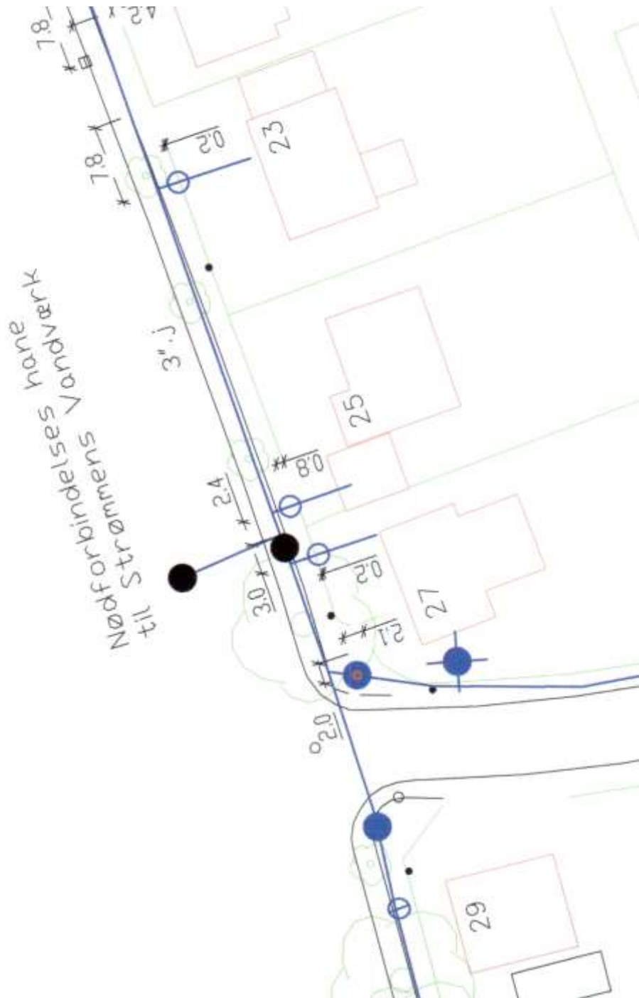
Figur 6.1 Nødforbindelsens placering på Valdemarsvej
